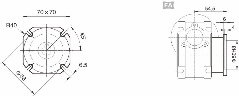
Output flange 输出法兰
